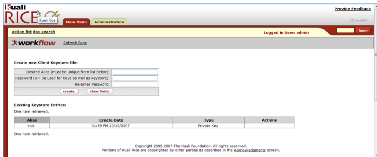
Figure 7.1. Create Keystore
