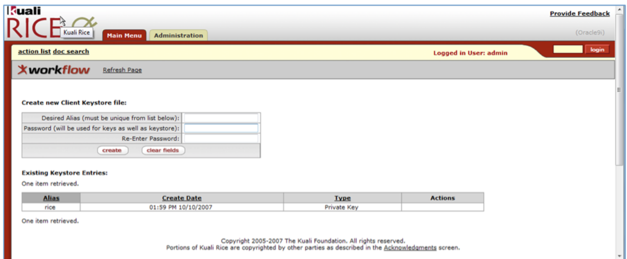
Figure 7.1. Create Keystore
